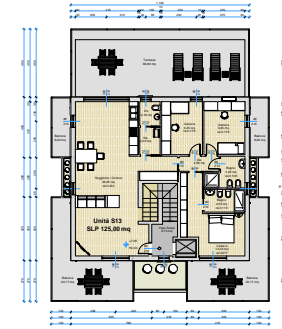
Pianta Piano Attico
