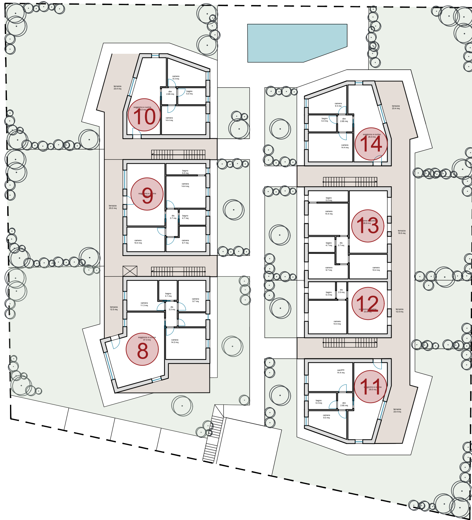
Planimetria piano primo - fuori scala
