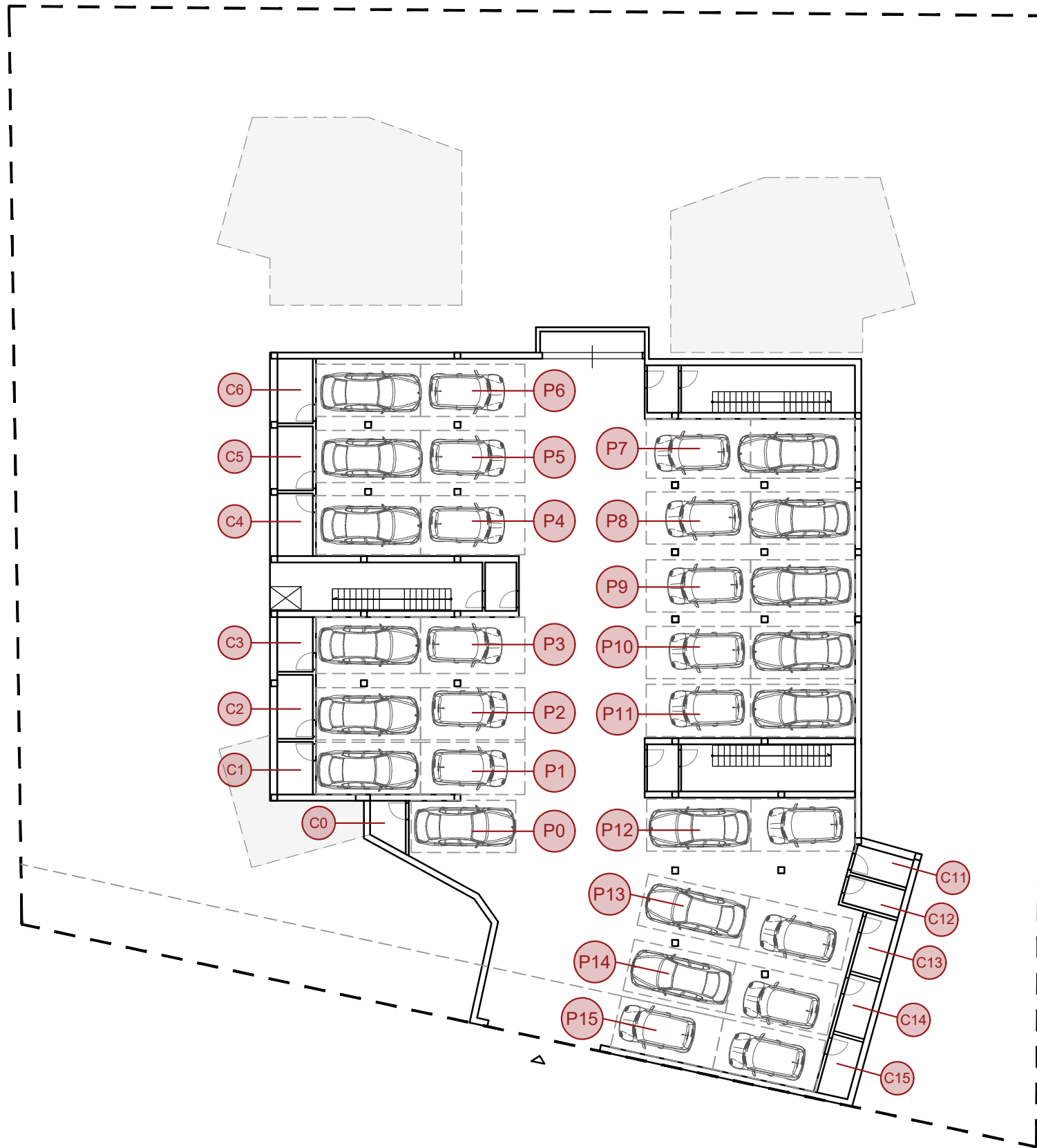
Planimetria piano interrato - fuori scala
